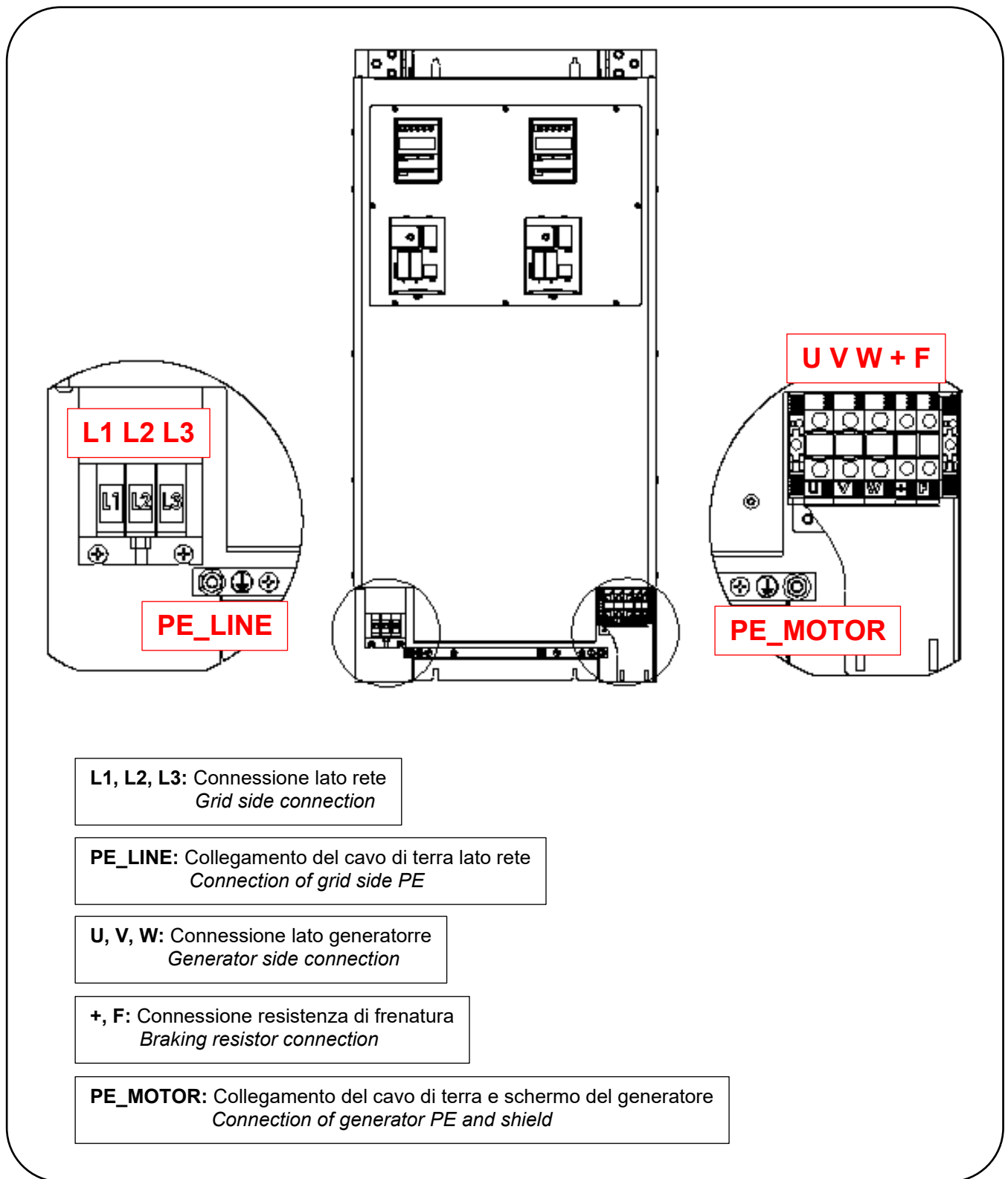
FIG. 17 - Collegamenti di potenza GE25, GE30 e GE40 / GE25, GE30 and GE40 power connections
