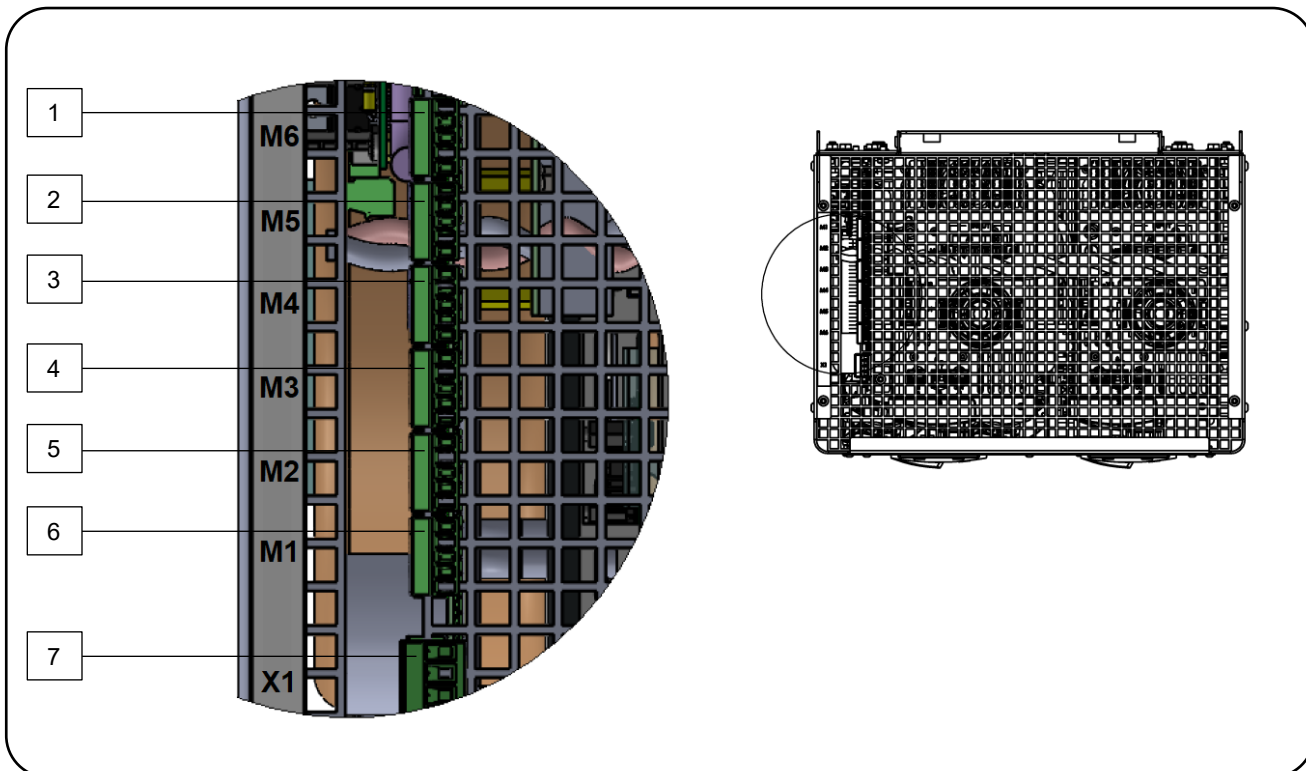
FIG. 9 – Pannello di controllo sulla parte superiore / Control panel on upper side
