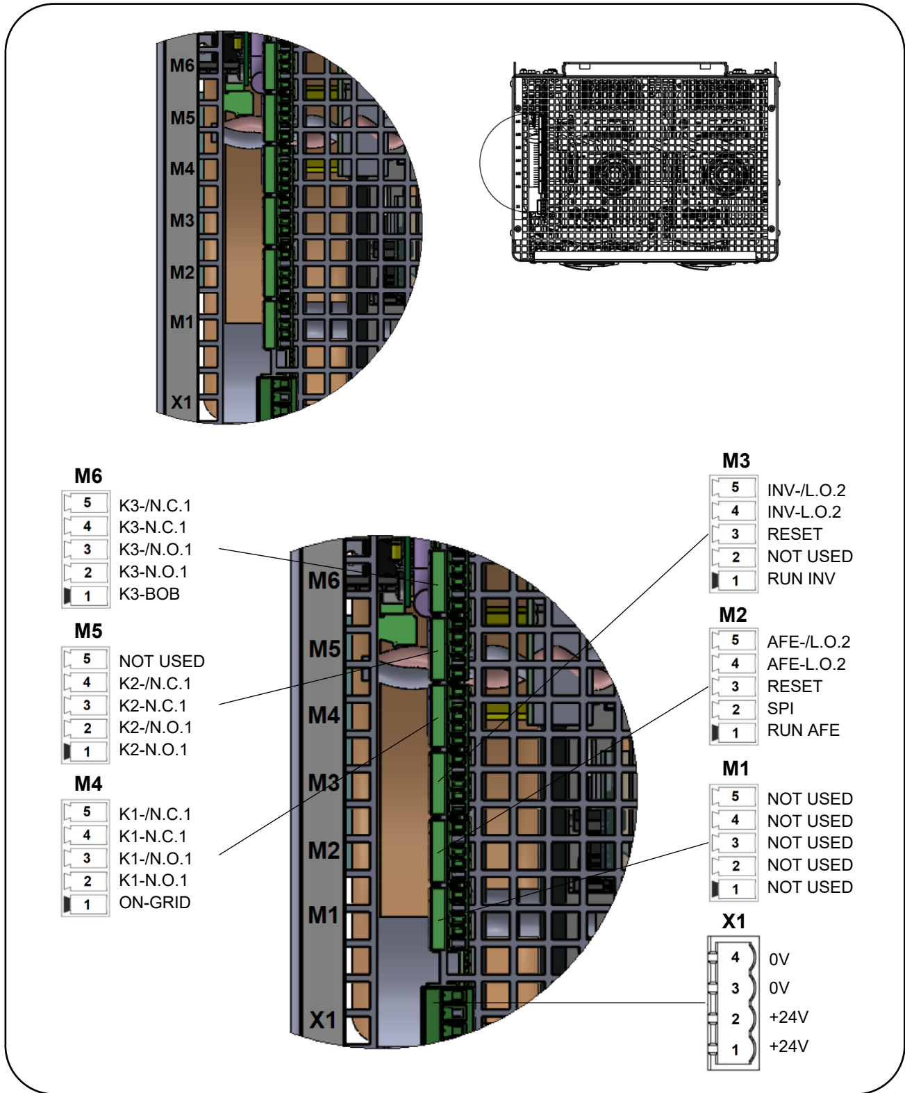
FIG. 19 -Collegamenti logici / Logic connections
